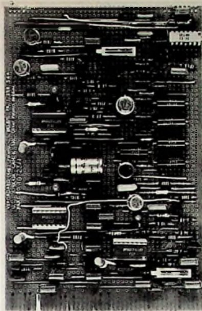
Kaart 2. exponentiële frequentiesturing voor de VCO (fig. 5)
